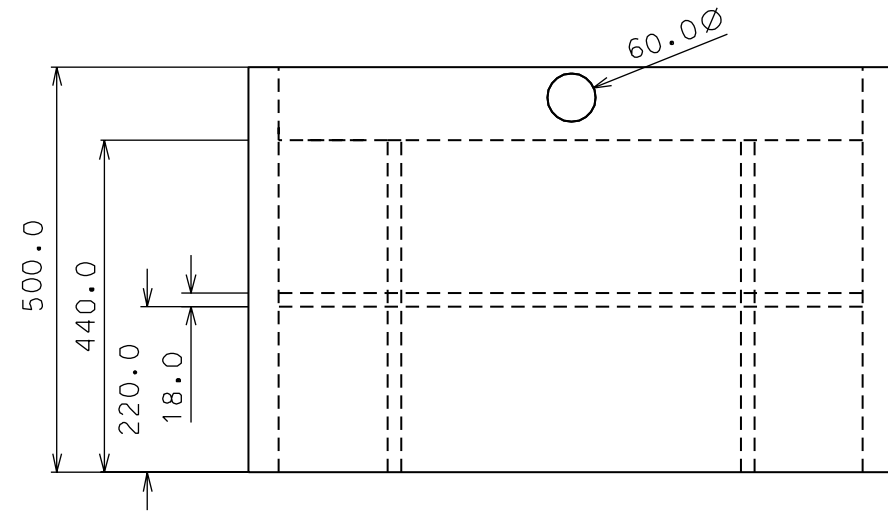
BOVENAANZICHT
