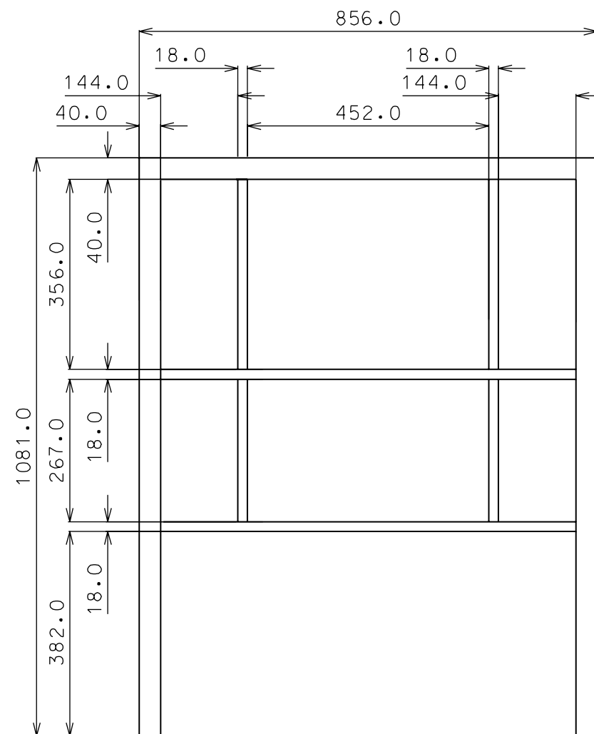
VOORAANZICHT
